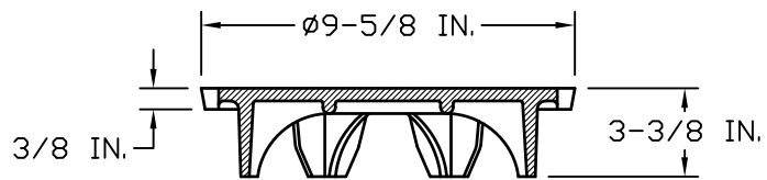
LID DETAIL
