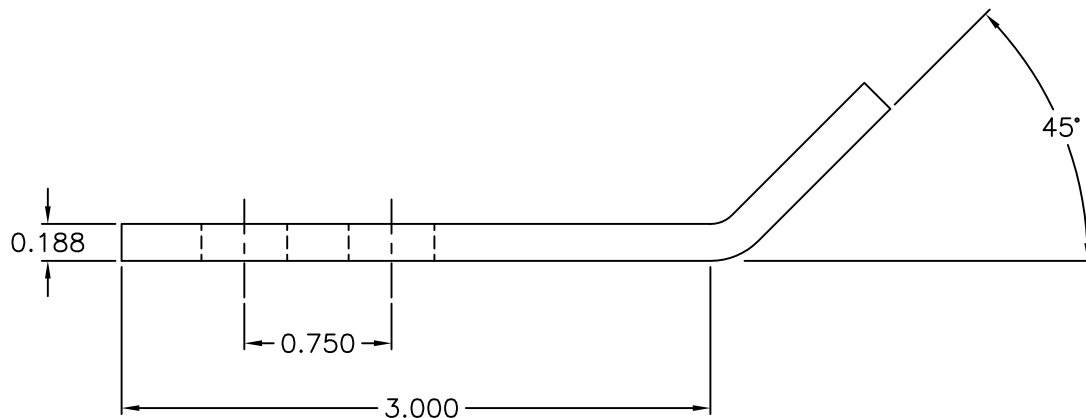
TINNED WELD LUG
