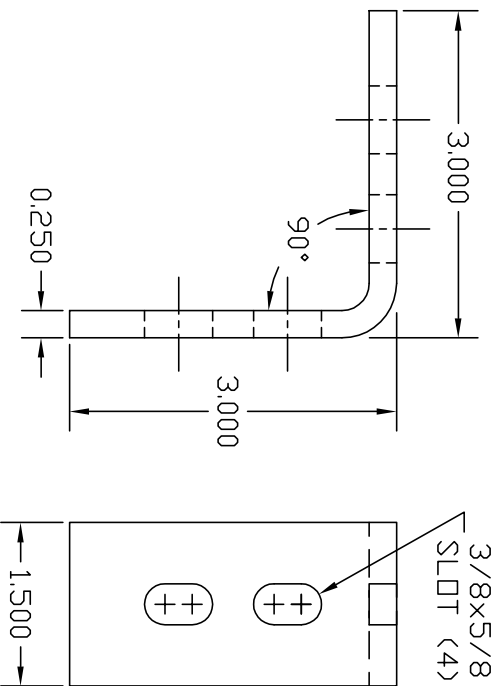
CU ELBOW 90°
