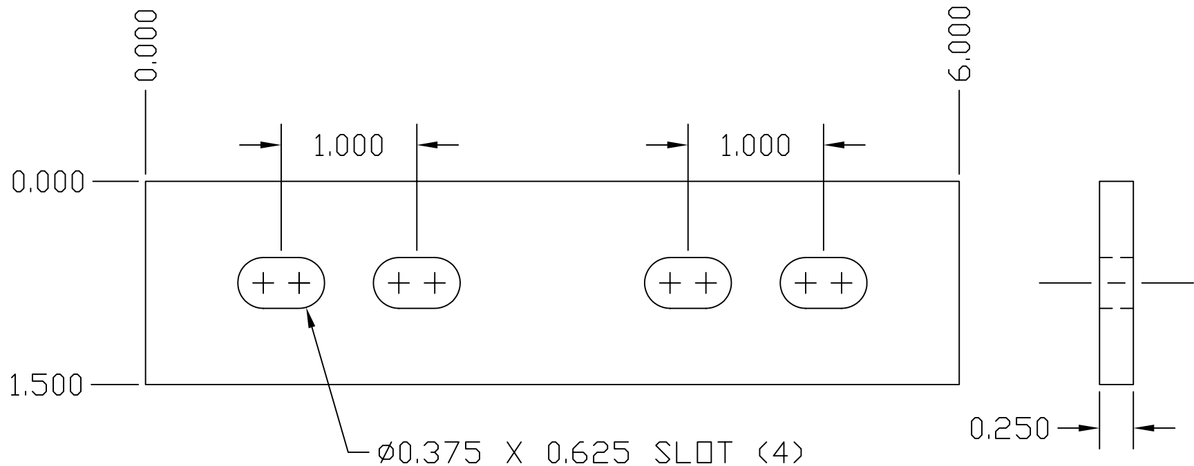
CU SPLICE PLATE
