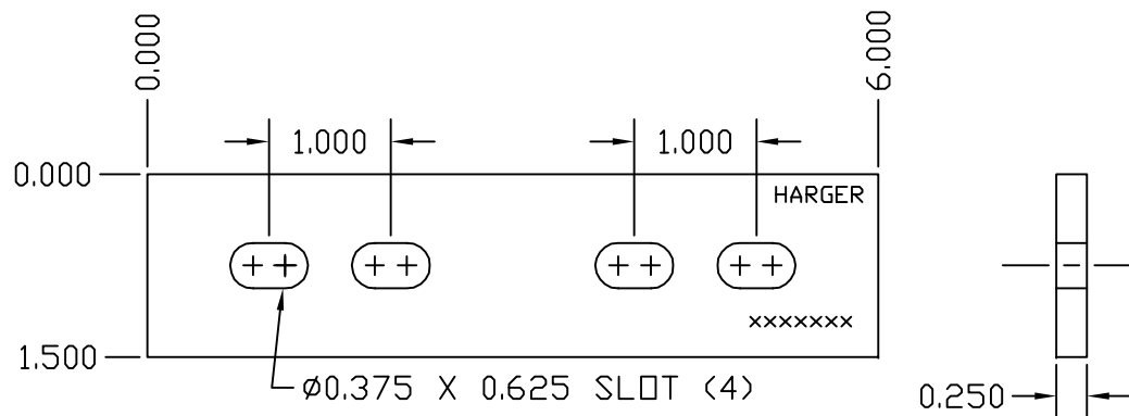
CU SPLICE PLATE
