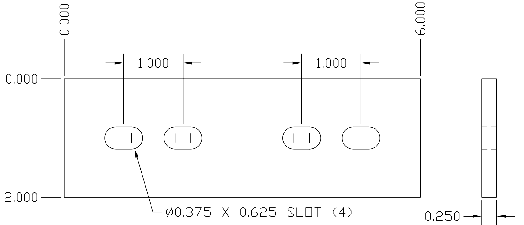
CU SPLICE PLATE
