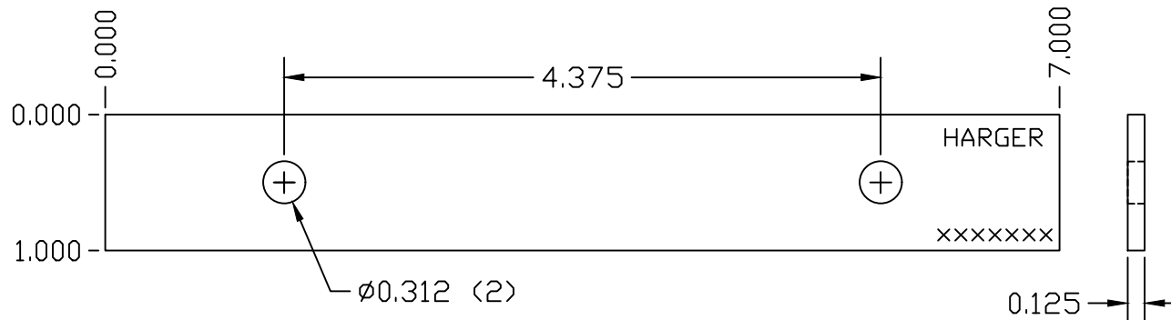
TOP CLAMP
