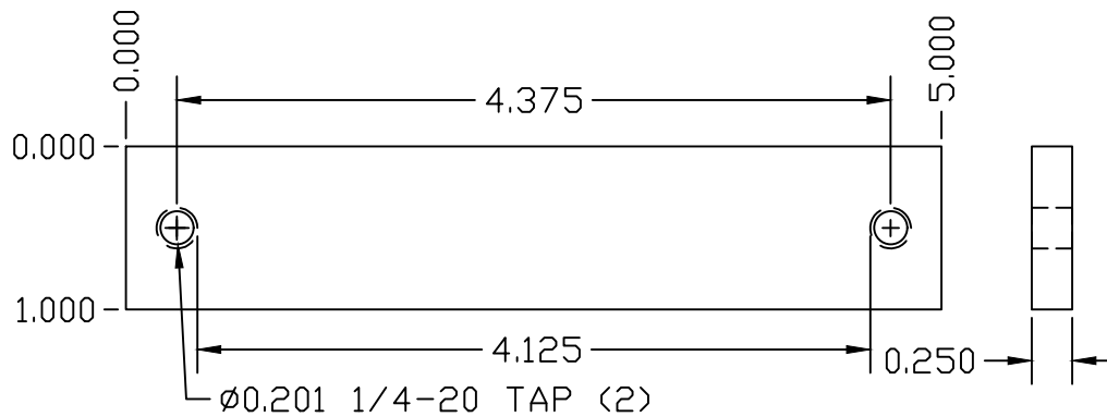
BOTTOM CLAMP
